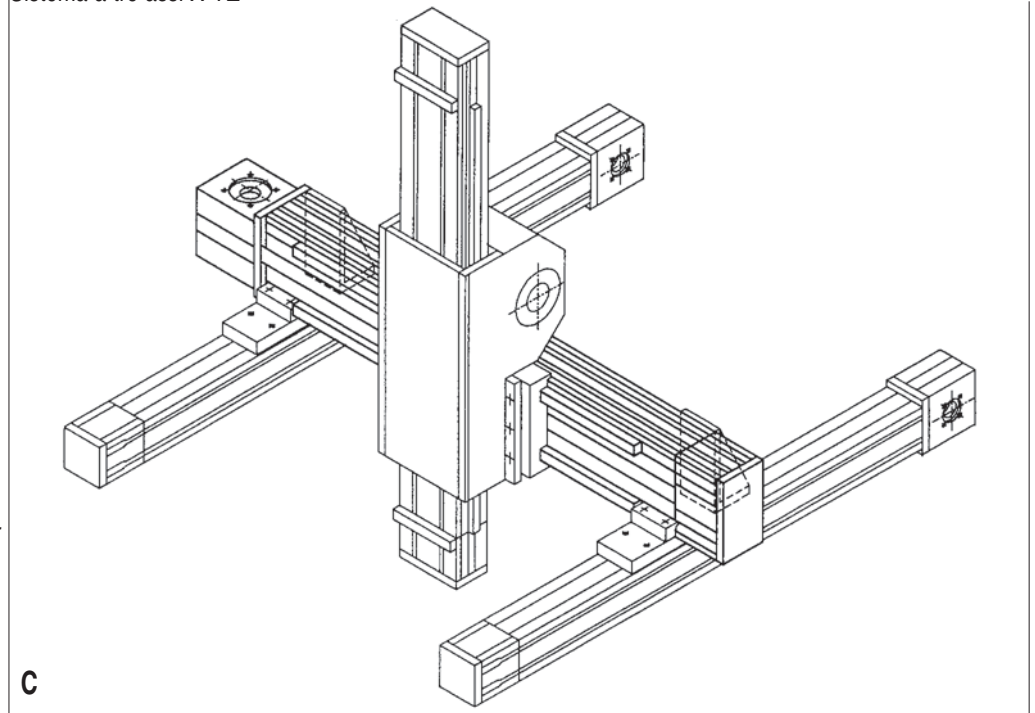
Systema a tre assi X-YZ
