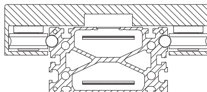
ROBOT 160 CE
